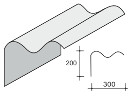
E příložník boční - přesah 200mm
