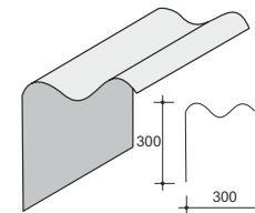
D příložník boční - přesah 300mm
