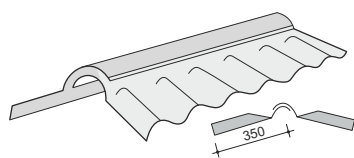
A hřebenáč profilovaný (pár)
