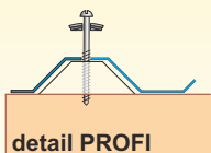
Polykarbonátový trapéz TR 76/16 - příklad detailu
